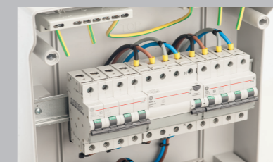
Ihned připraveno k instalaci, PE/N svorkovnice součástí Ready to install the terminal blocks for neutral and earth connection
