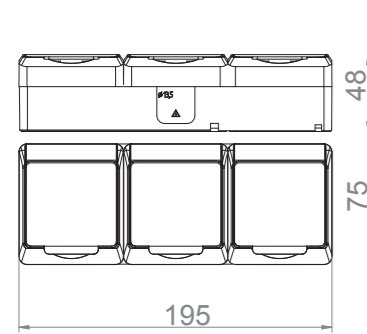
Zásuvka s ochranným kolíkem
