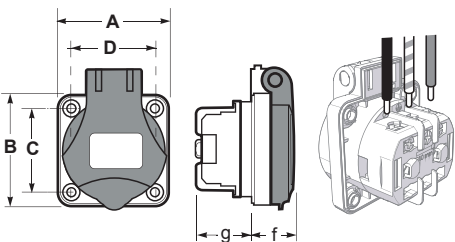
Vestavné zásuvky IP54 / Panel sockets IP54
