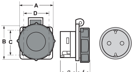
Vestavná zásuvka IP68 / Panel plug IP68
