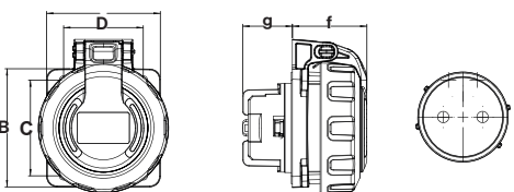
Vestavná zásuvka IP68 / Panel plug IP68
