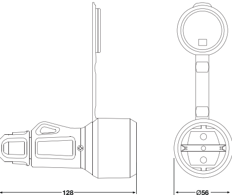
Spojky s gumovou krytkou a s ochranným kolíkem IP54 / Mobile socket 2P+T 16A 250V FR detachable IP54 - Obj.č. / Item 2165F
