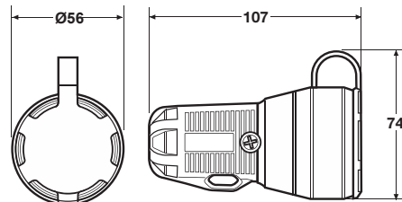
Rozměry v mm / Dimensions in mm
