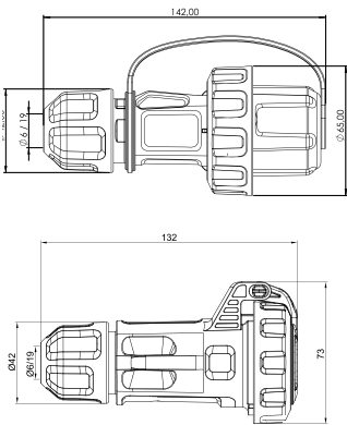
Vidlice IP68 - spojky IP67 / Plug IP68 - Socket IP67
