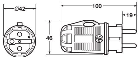
Gumové vidlice IP54 / Rubber plug IP54 - Obj.č. / Item 1167
