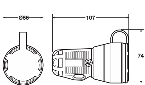
Gumové spojky IP54 / Rubber socket IP54 - Obj.č. / Item 2167
