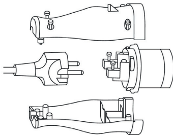
Adaptér domovní - průmyslový PLUG SHELL IP20/44 / Domestic-industrial PLUG SHELL IP20/44
