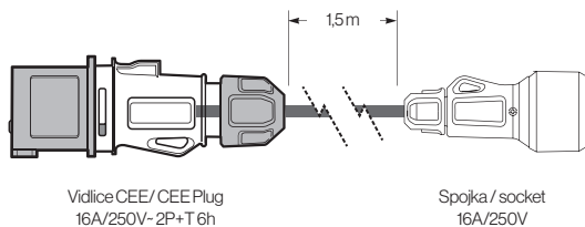
Adaptér průmyslový - domovní IP54 / Industrial-domestic IP54
