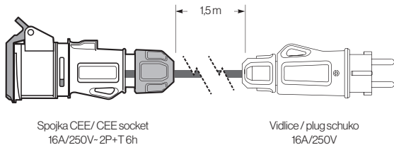
Adaptér průmyslový - domovní IP54 / Industrial-domestic IP54
