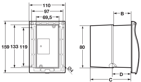
Výklopná napájecí vidlice pro karavany IP44 / Fush mounting plug for caravan IP44
