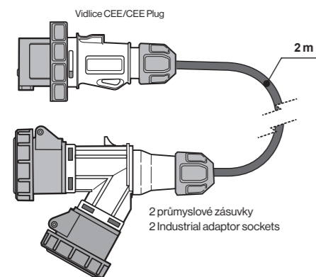
Vícenásobný adaptér s kabelem IP67 Industrial adaptors 2 ways IP67
