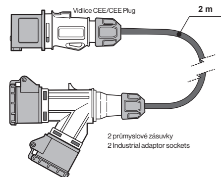
Vícenásobný adaptér s kabelem IP54 Industrial adaptors 2 ways IP54
