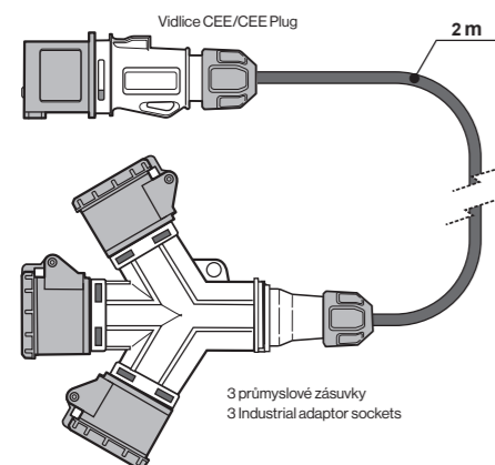
Vícenásobný adaptér s kabelem IP54 Industrial adaptors 3 ways IP54
