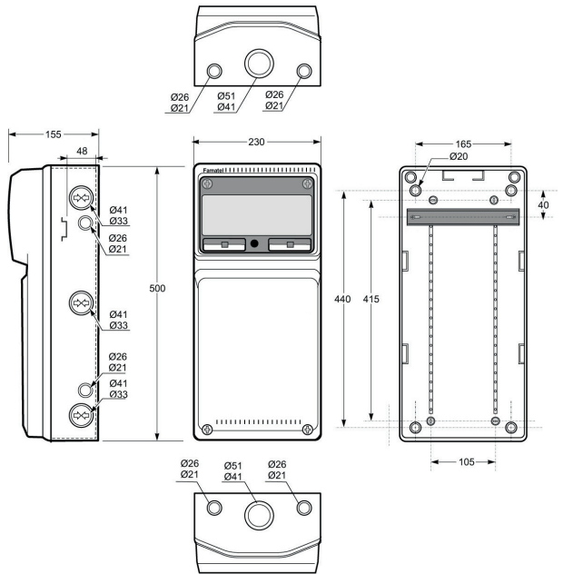
Rozvodnice AcquaCOMBI / Blind box - Obj. č. 3951
