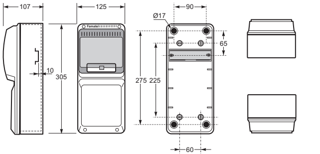
Rozvodnice AcquaCOMBI / Blind box - Obj. č. 3927
