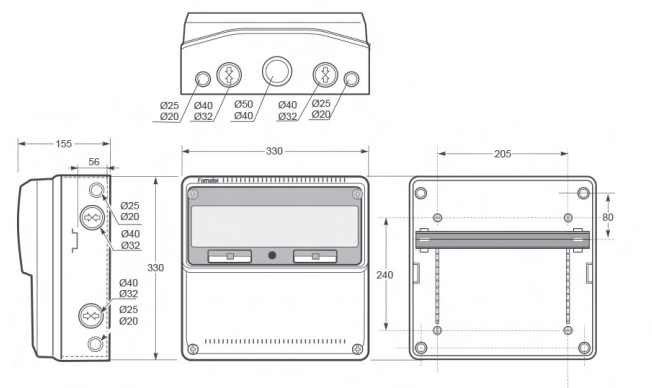
Rozvodnice AcquaCOMBI / Blind box - Obj. č. 3952
