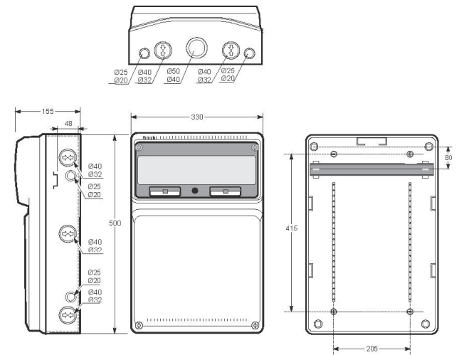
Rozvodnice AcquaCOMBI / Blind box - Obj. č. 3977
