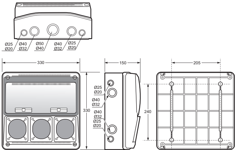
Rozvodnice AcquaCOMBI / Knock-out box - Obj.č. 3975
